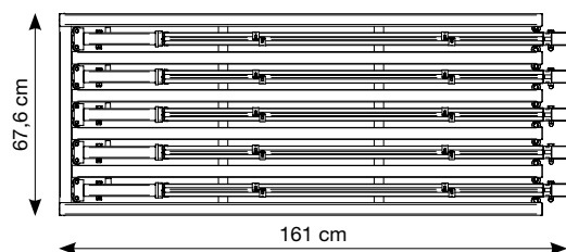
Pianta
